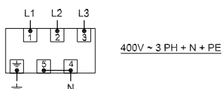
SCHEMA COLLEGAMENTO MORSETTIERA A 5 + 1 POLI
